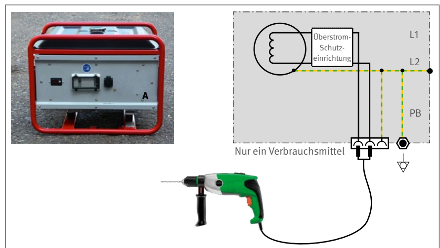
Abb. 6 Stromerzeuger ohne Erdungsanschluss mit nur einer Steckdose und nur einem angeschlossenen Verbrauchsmittel
